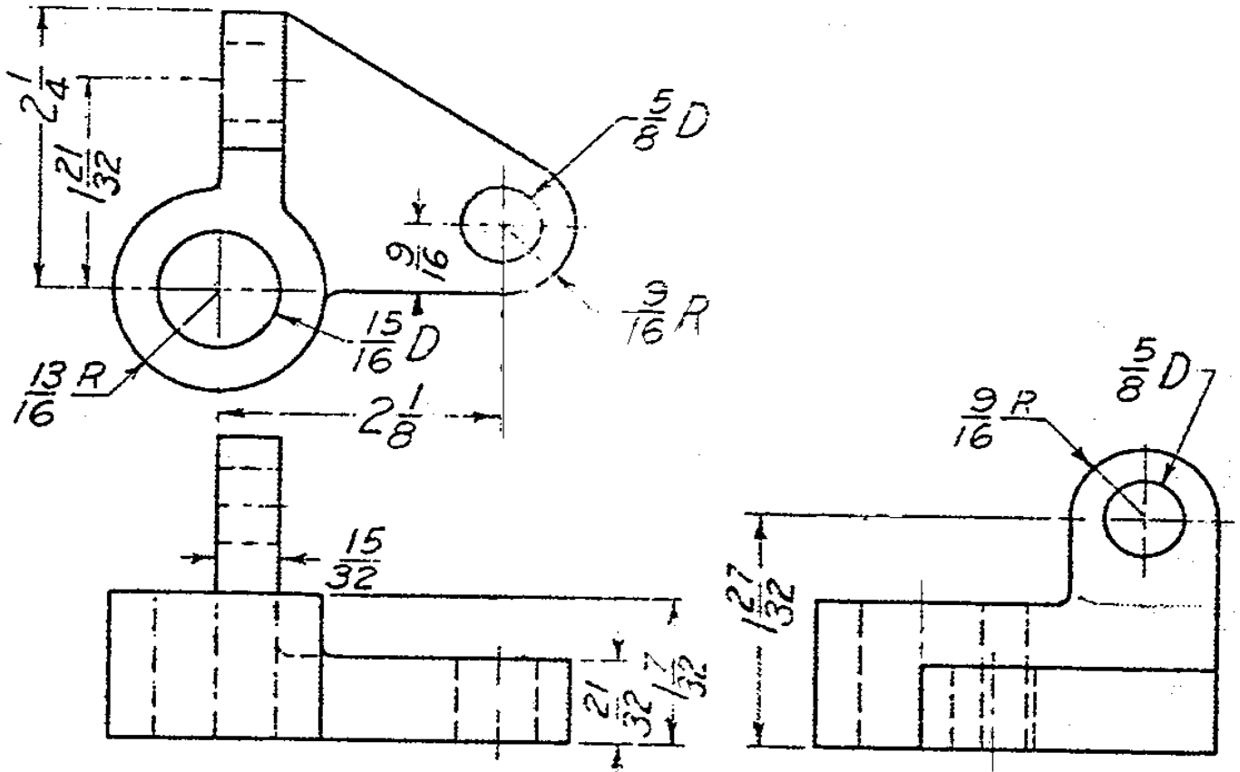
Prob. 5.1.10 Cable clip
